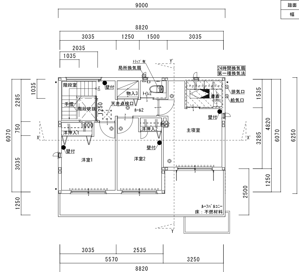
2階平面図
