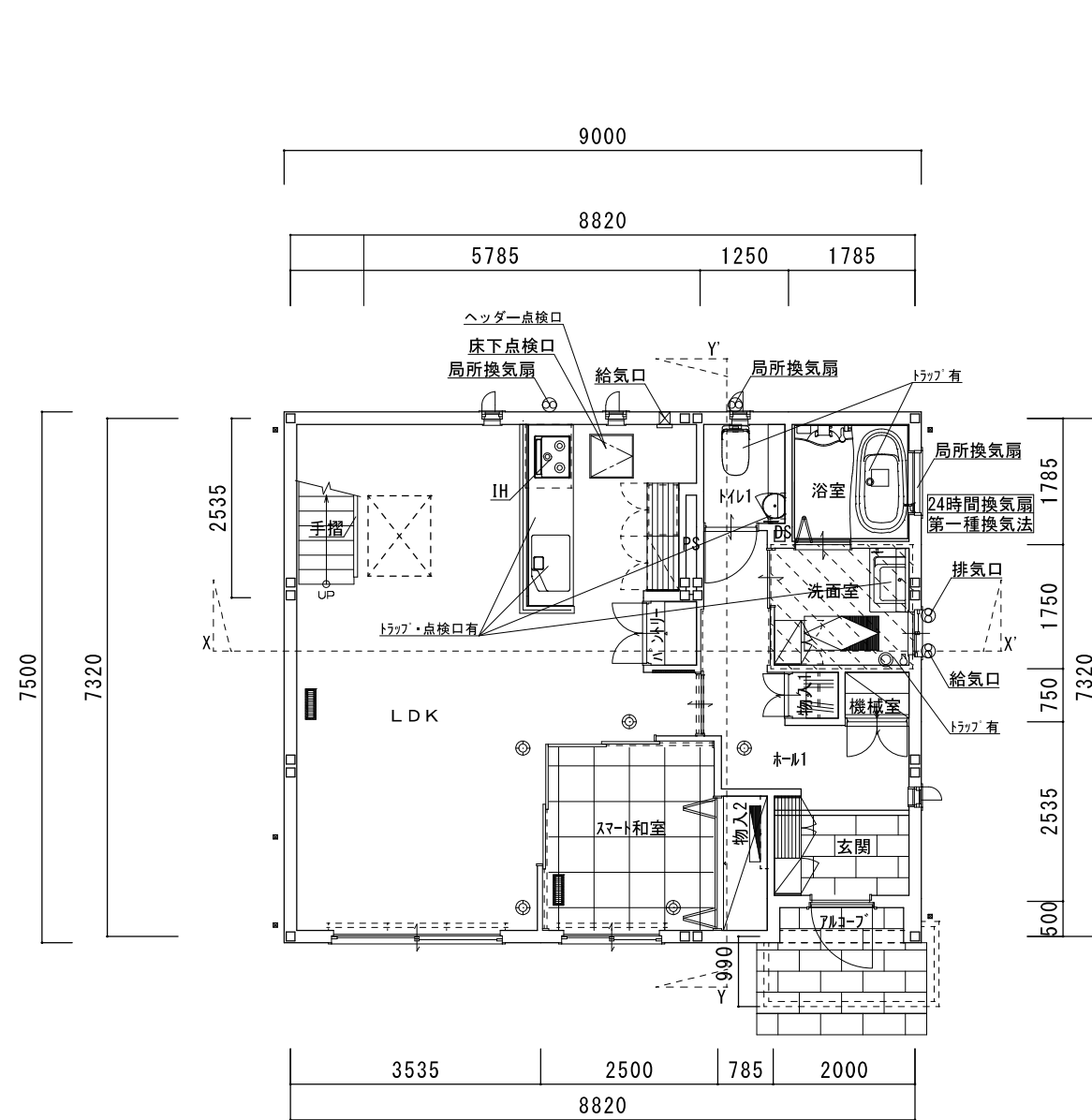
1階平面図
