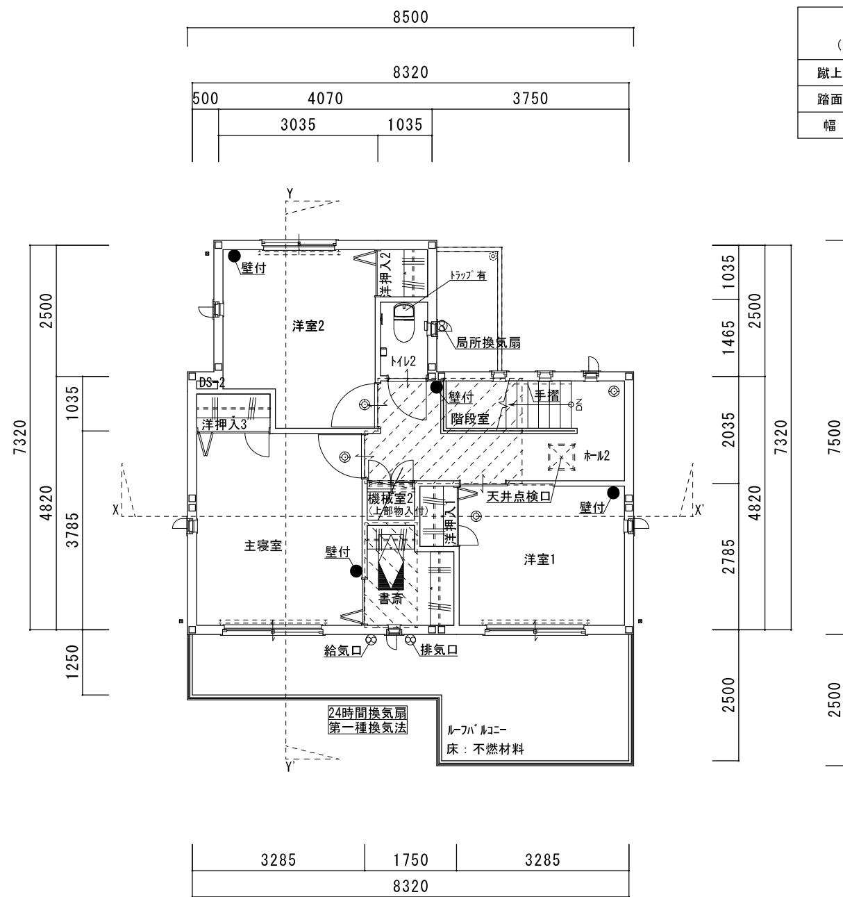
2階平面図
