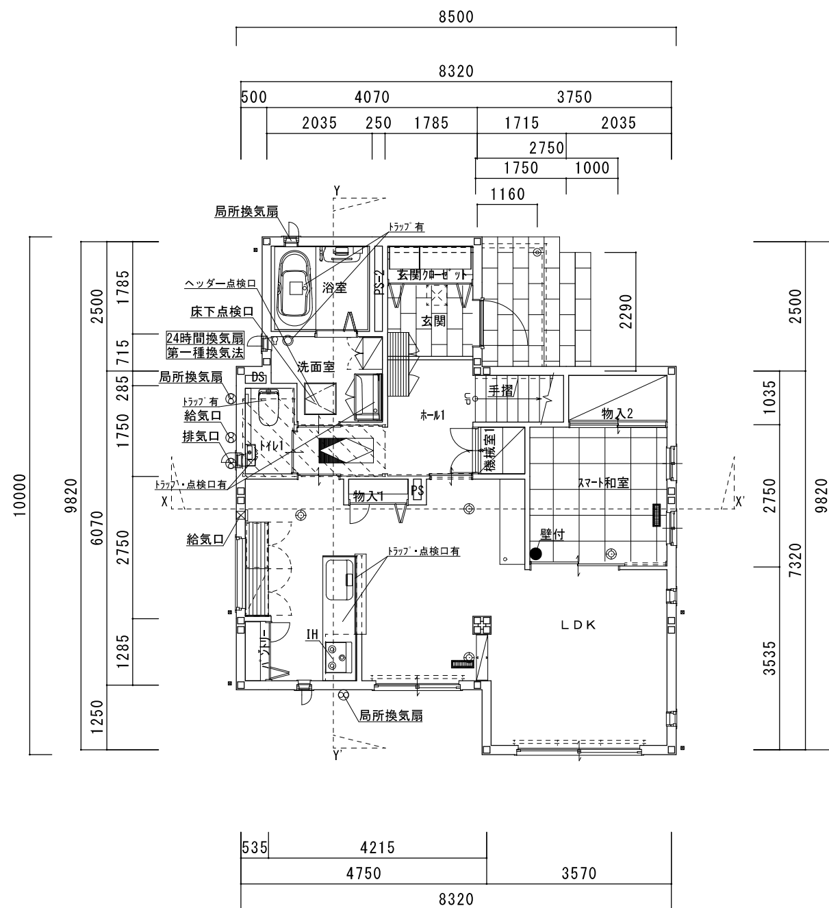
1階平面図
